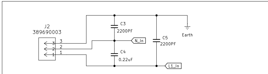
AC 1PH Input
